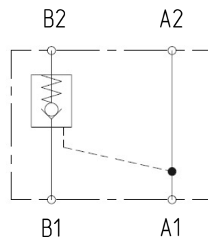
Схема гидравлическая
